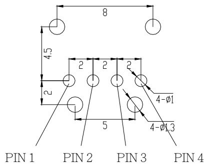
P.C.B LAND DIMENSION
